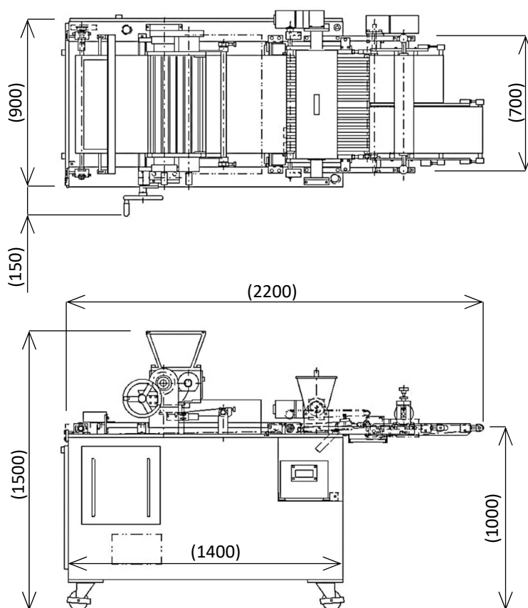
◆ 寸法図(一例) DIMENSION: mm
