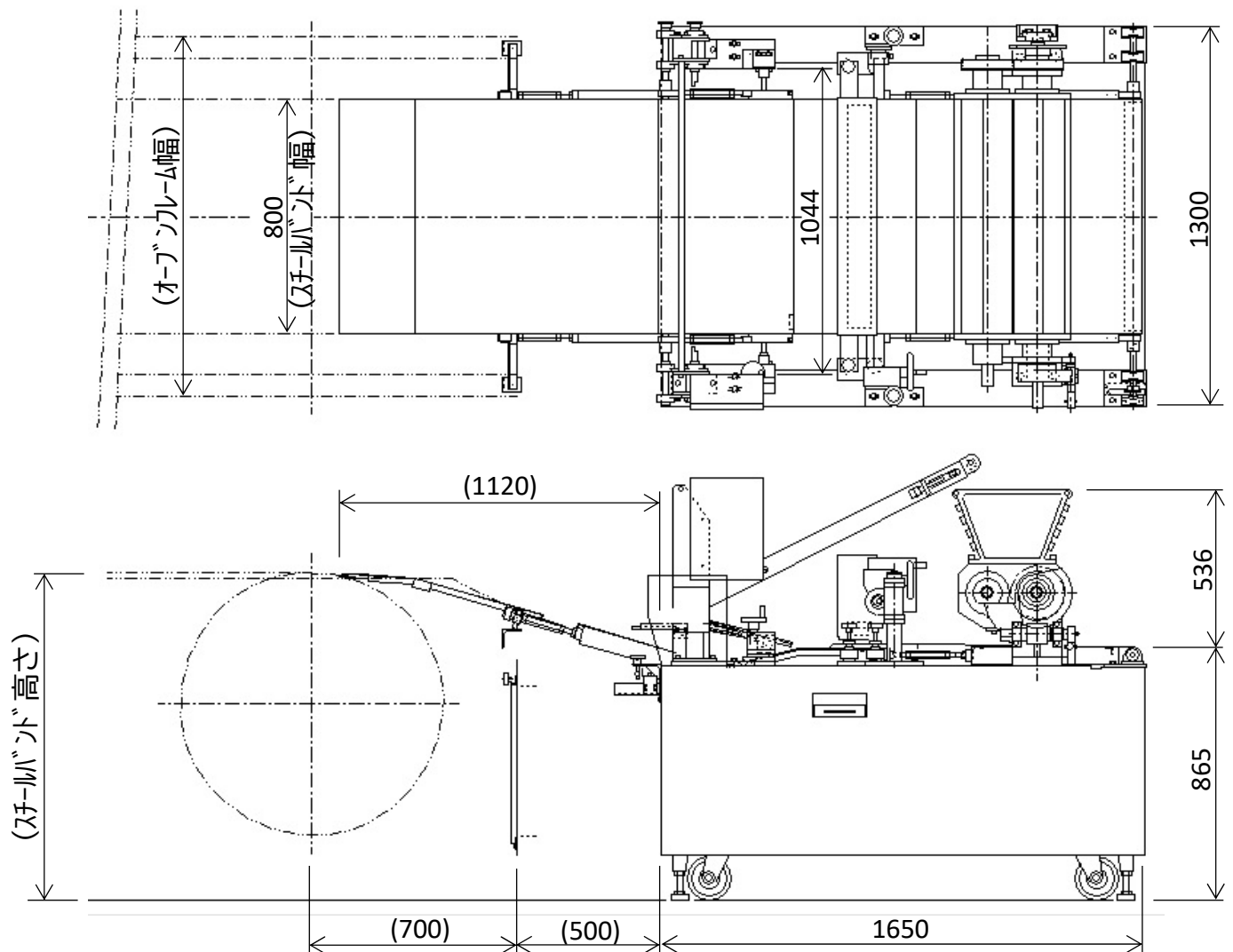
【800mm幅 上流設置仕様 参考図(mm)】
